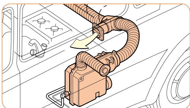
Truma E-kachels
