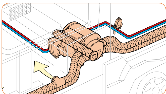
Truma Combi-verwarmingen
